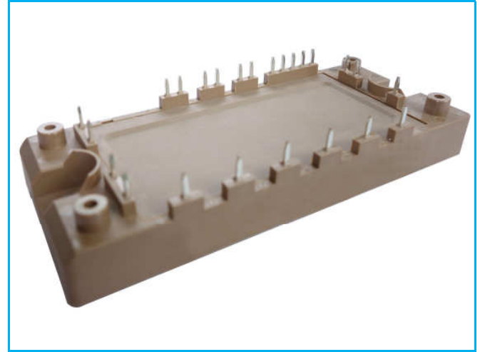
Rectifier+Brake+Inverter
