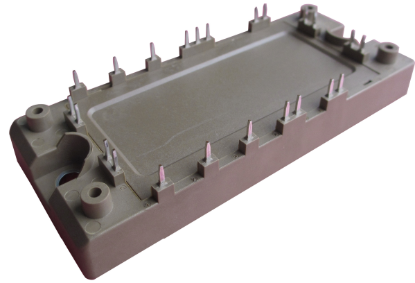
Rectifier+Brake+Inverter
